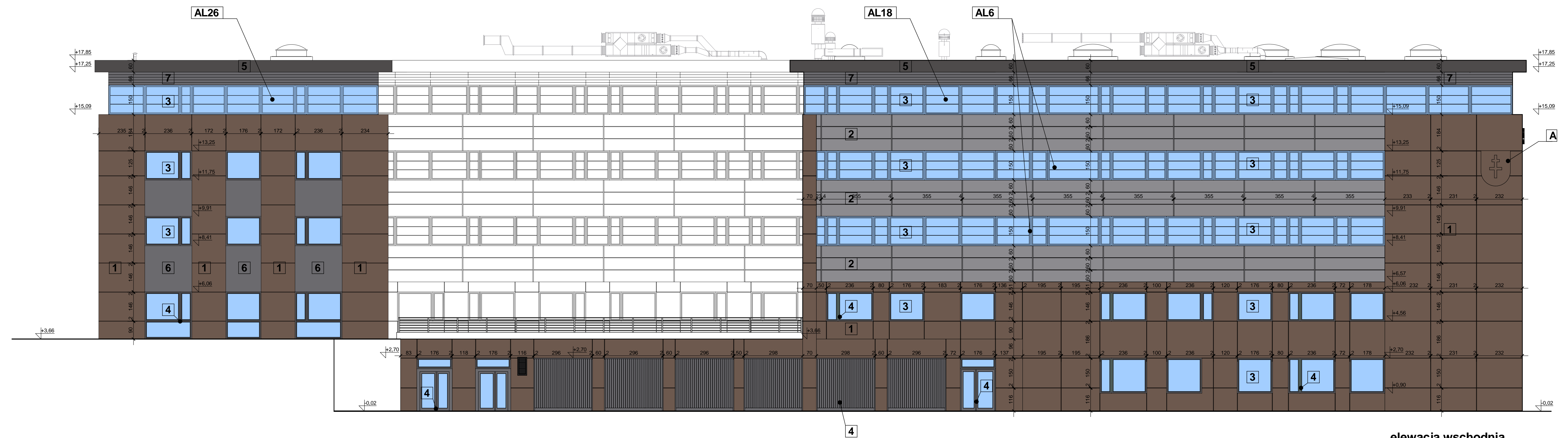
elewacja wschodnia
